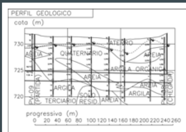
Figura 5 - Perfil geológico longitudinal entre PV9 e PV8
