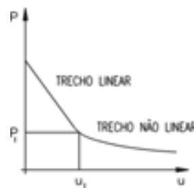
Figura 4 - Curva de reação do macijo para comportamento elasto-plástico
